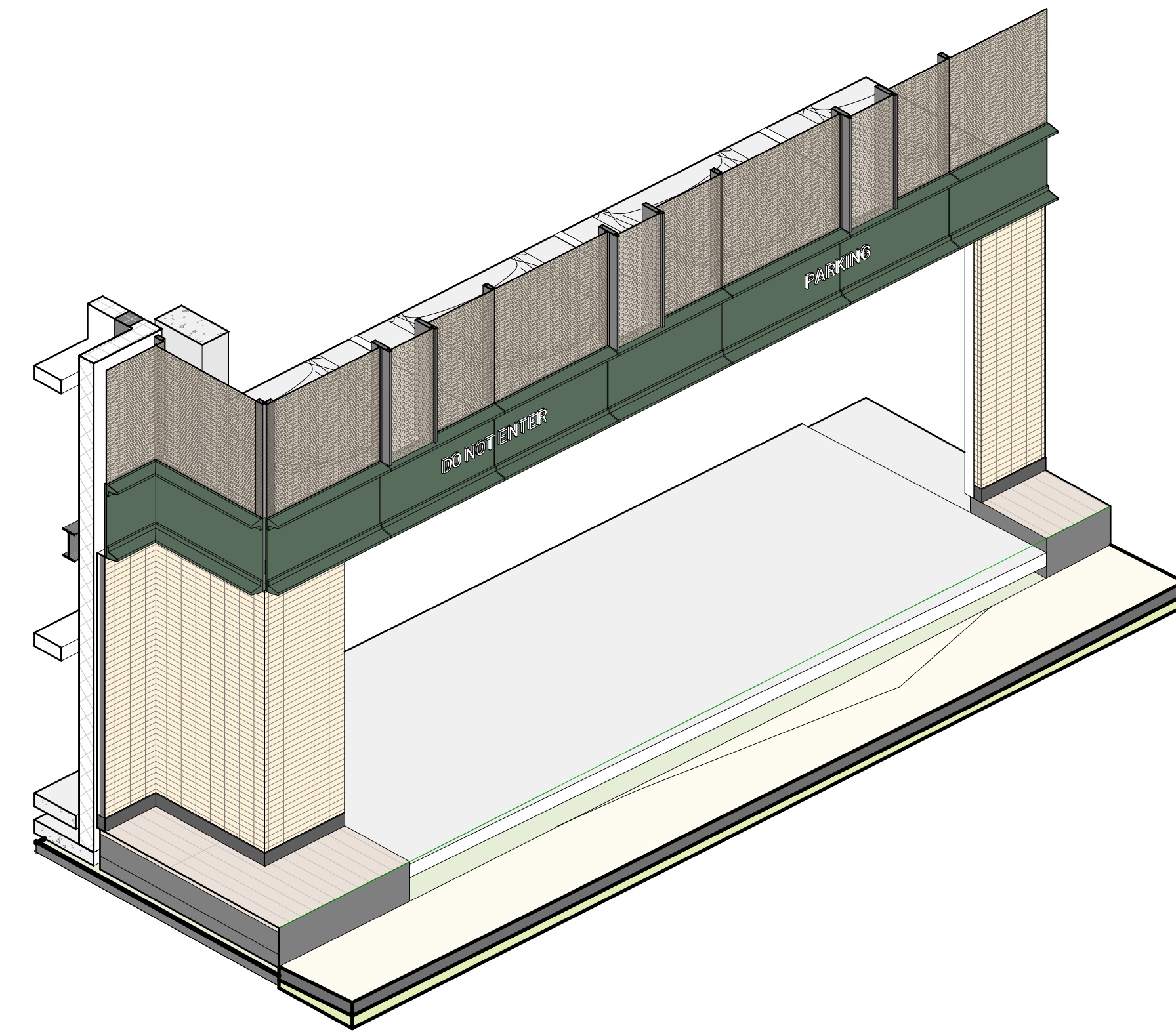
4 AXONOMETRIC
